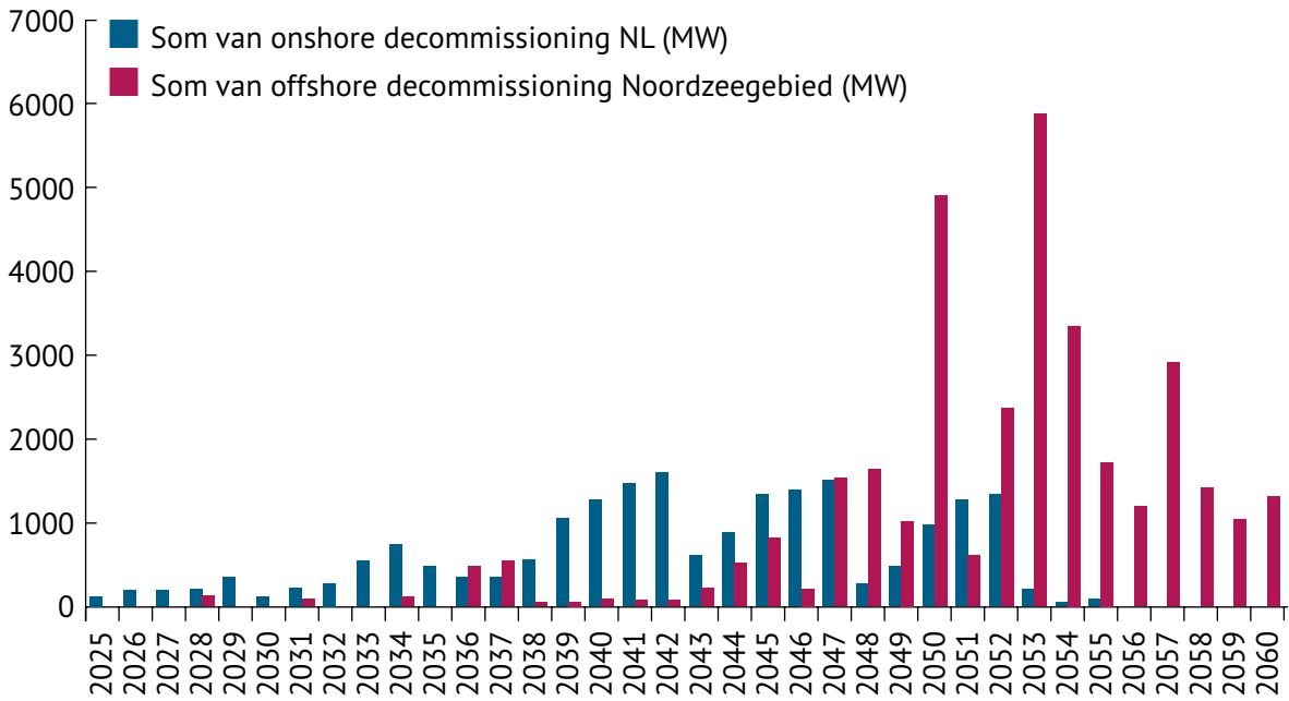
Figuur 7: Grafiek waarin over tijd wordt aangegeven hoeveel windturbines moeten worden ontmanteld voor zowel onshore als offshore.
